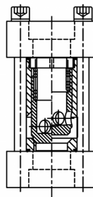
CETOP Flanges
