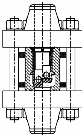
ANSI Flanges
